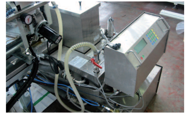
Vasca colla con pre-fusore completa di viscosimetro Glue tank with glue melter and viscosity control device Bac à colle avec chaudière douée de viscosimètre 配粘度计的涂胶预熔胶料盒
